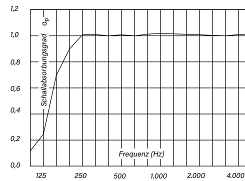
Screen50 Deckenabsorber - abgehängt 400 - 1500 mm Deckenabstand
