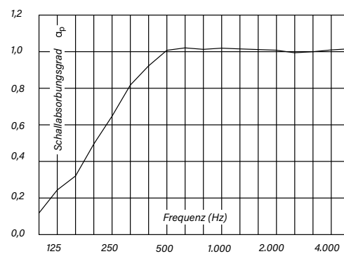
Screen50 Deckenabsorber - direkt montiert 20 mm Deckenabstand
