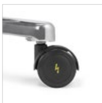
Weiche, lastabhängig gebremste Rollen für harte Böden, leitfähig (Ø 50 mm, abgedeckt) Soft, load-dependent locking castors for hard floors, conductive (Ø 50 mm, with cover caps) (R70HGSL) Harte Rollen | Hard castors (R70HGSL)
